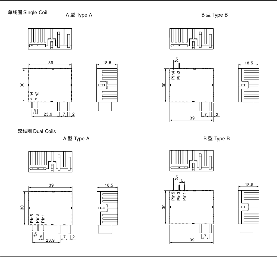
外形尺寸 PROFILE DIMENSION
