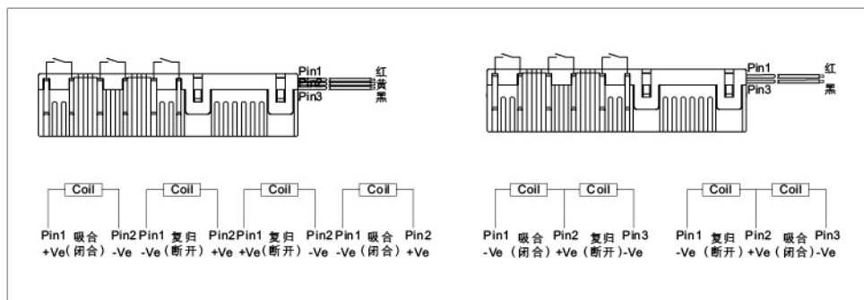
接线图
