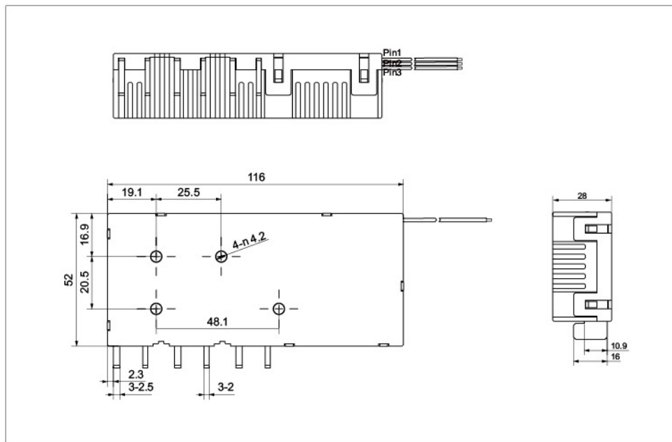
外形尺寸图
